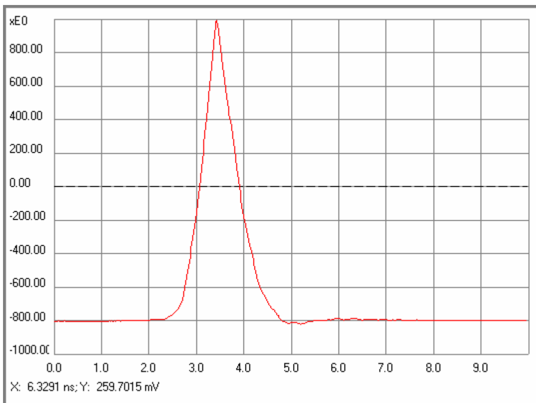
по оси X – 1 нс/дел; по оси Y – 20 В/дел с учетом ослабления 40 дБ
