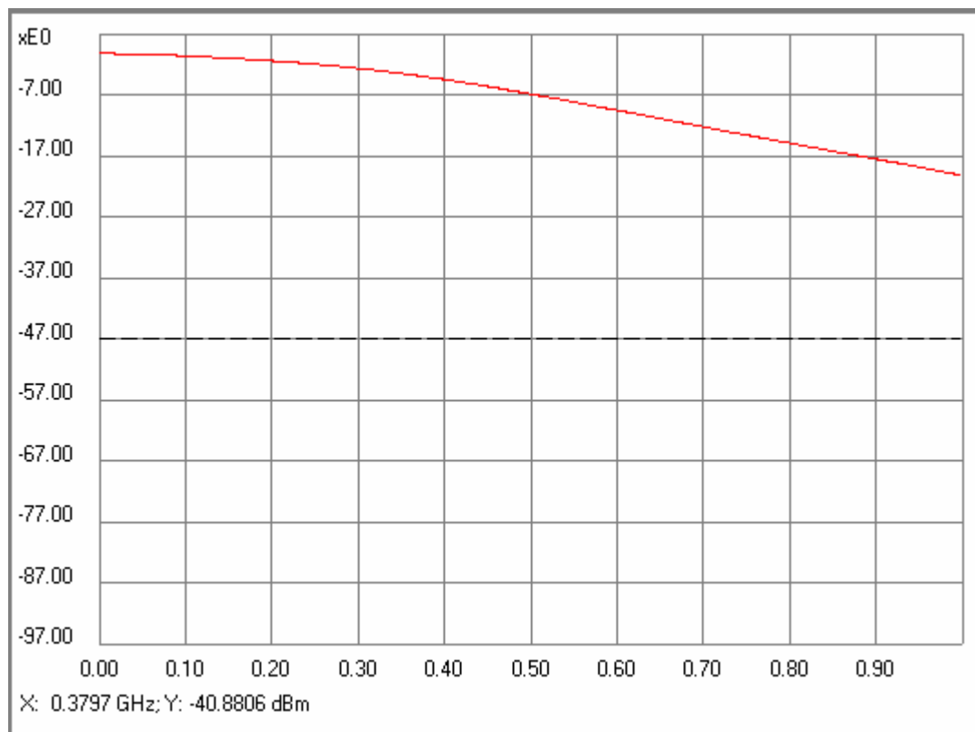
по оси X – 0,1 ГГц/дел; по оси Y – 10 дБм/дел
