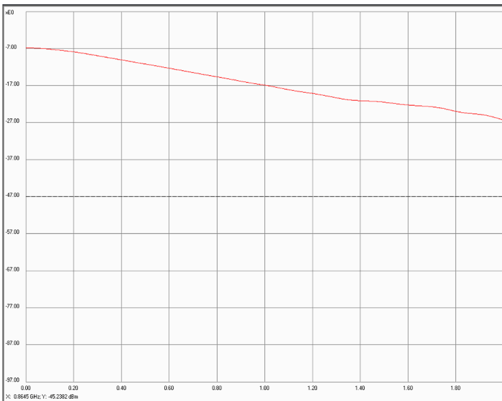
по оси X – 0,2 ГГц/дел; по оси Y – 10 дБм/дел
