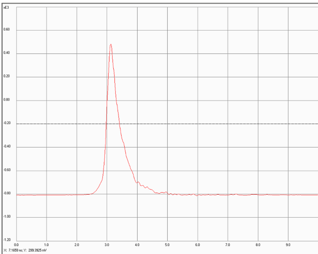
по оси X – 1 нс/дел; по оси Y – 20 В/дел с учетом ослабления 40 дБ
