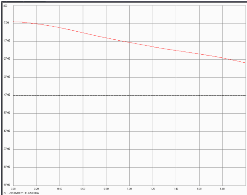
по оси X – 0,3 ГГц/дел; по оси Y – 10 дБм/дел
