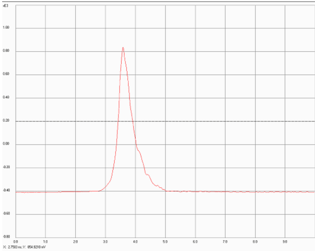
по оси X – 1 нс/дел; по оси Y – 20 В/дел с учетом ослабления 40 дБ
